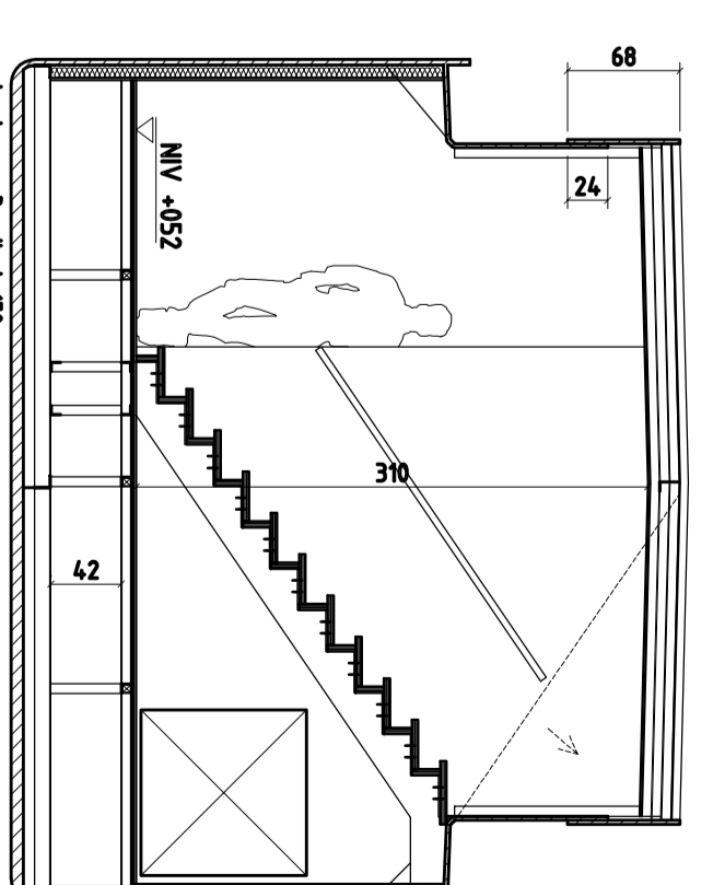
COUPE DD
